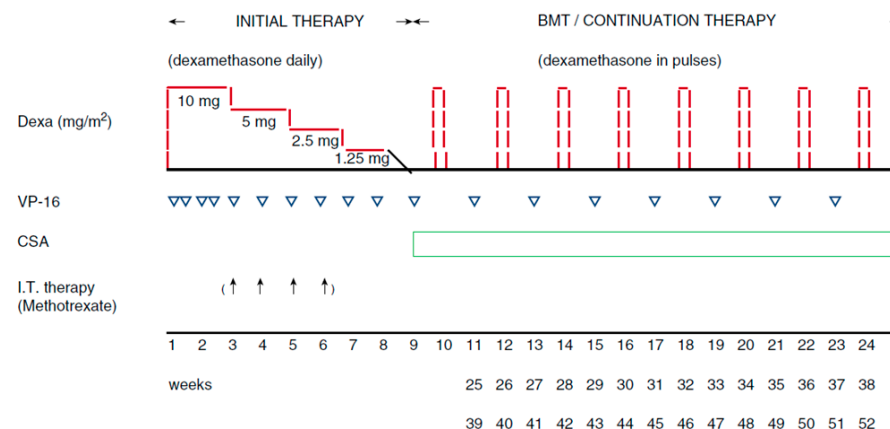
Obrázek 3. Protokol HLH-94.
